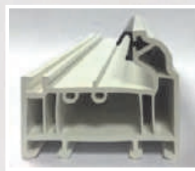
56mm PVCu
